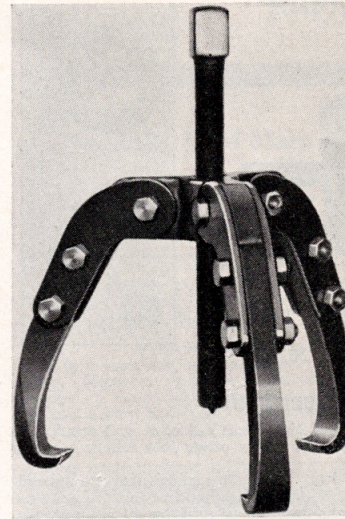
No. 2025-A 3-Jaw Puller
